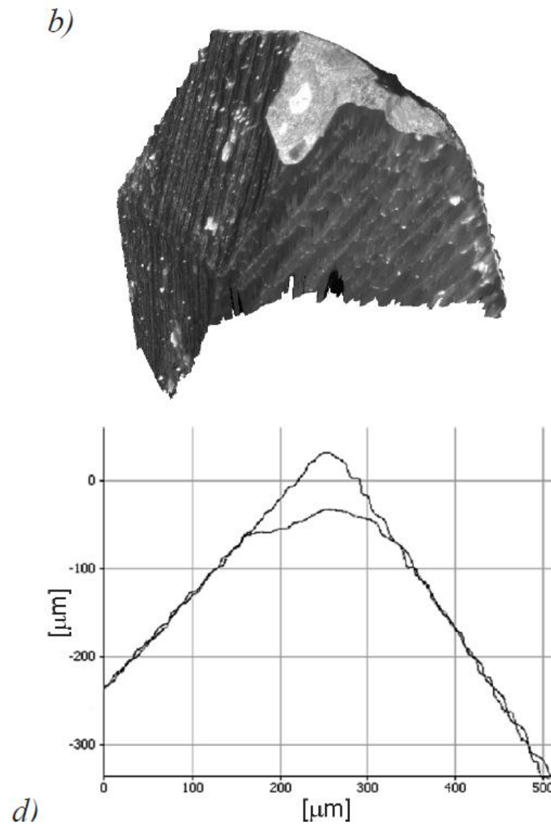
Merenje pohabanosti rezne ivice glodala, a) nepohabana rezna ivica, b) pohabana rezna ivica, c) zapreminska razlika između pohabane i nepohabane rezne ivice, d) kopracija profila
