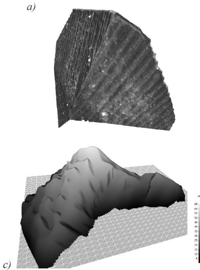
Merenje pohabanosti rezne ivice glodala, a) nepohabana rezna ivica, b) pohabana rezna ivica, c) zapreminska razlika između pohabane i nepohabane rezne ivice, d) kopracija profila
